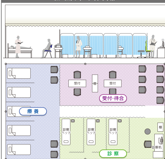
3k×5kテント レイアウト案
